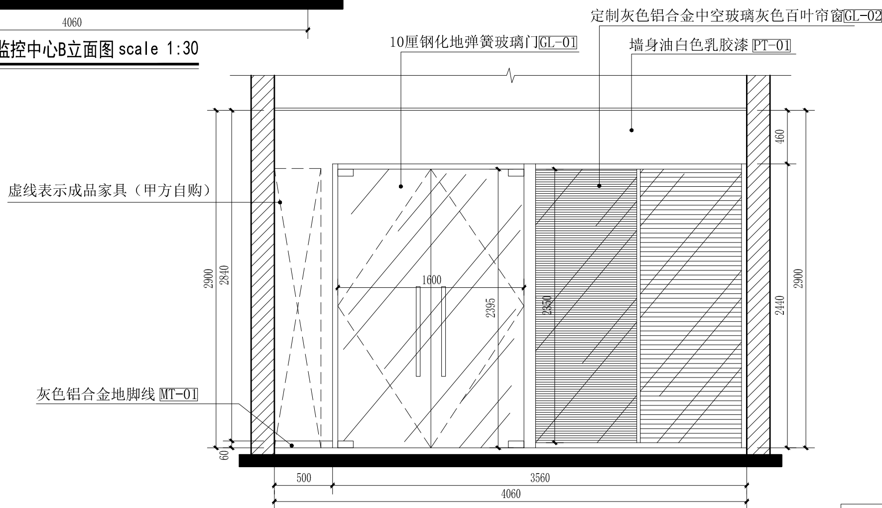
运调监控中心D立面图 scale 1:30
