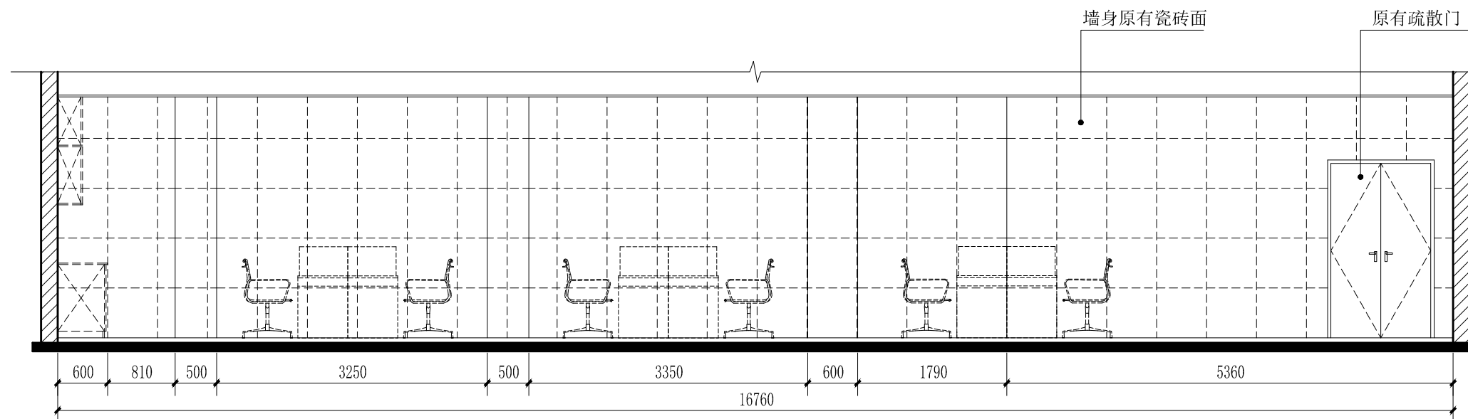
车载监控中心C立面图scale 1:60
