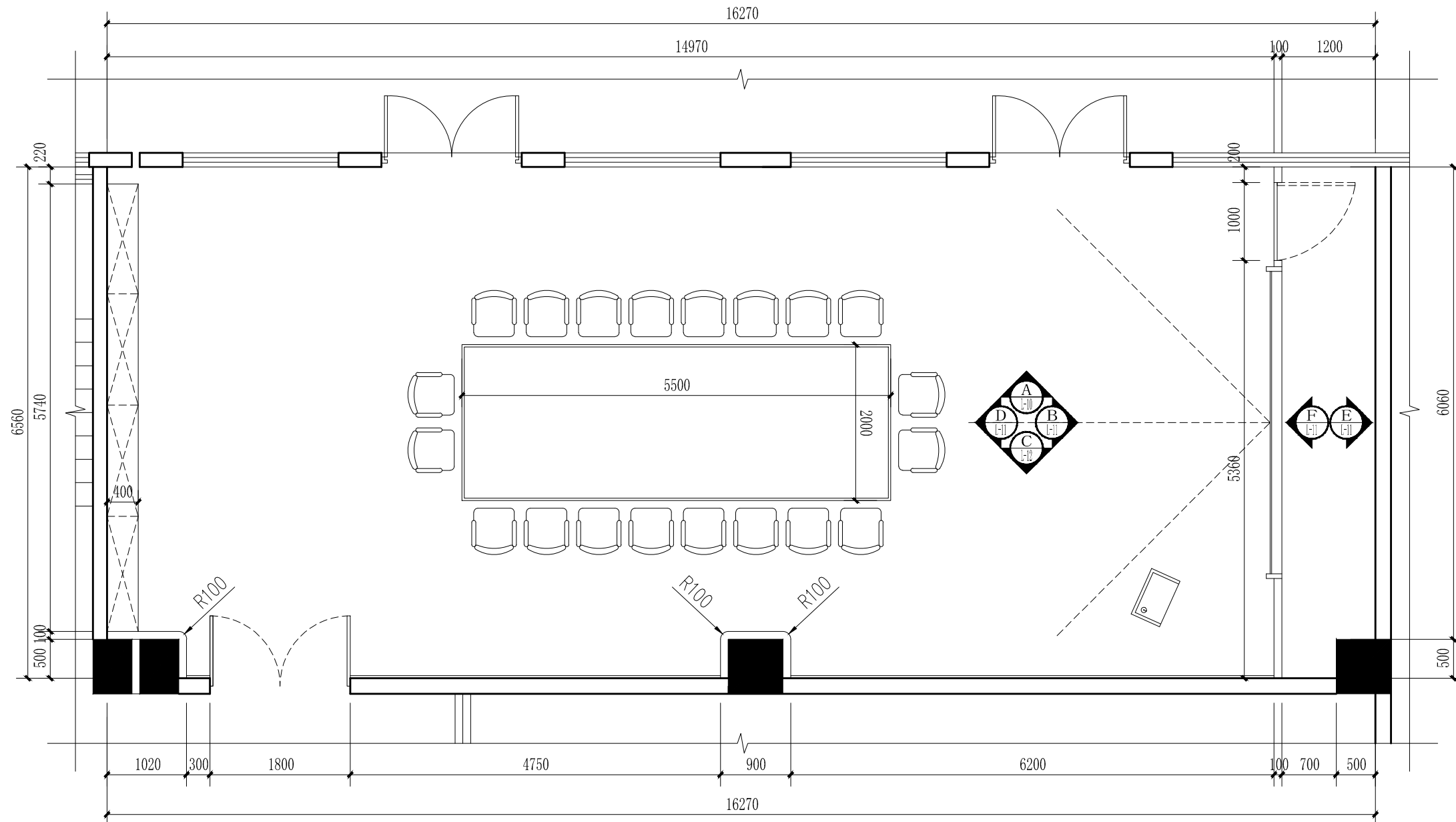
智能调度大厅平面图 scale 1:60
