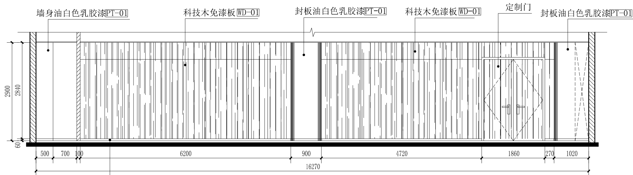
智能调度大厅C立面图scale 1:60
