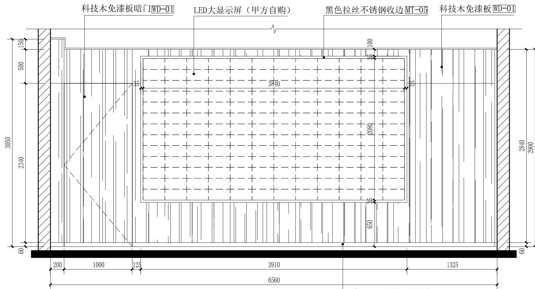
智能调度大厅B立面图 scale 1:30
