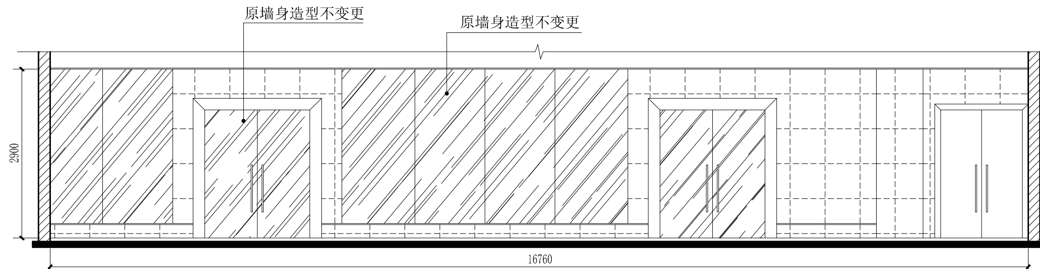
车载监控中心A立面图scale 1:60
