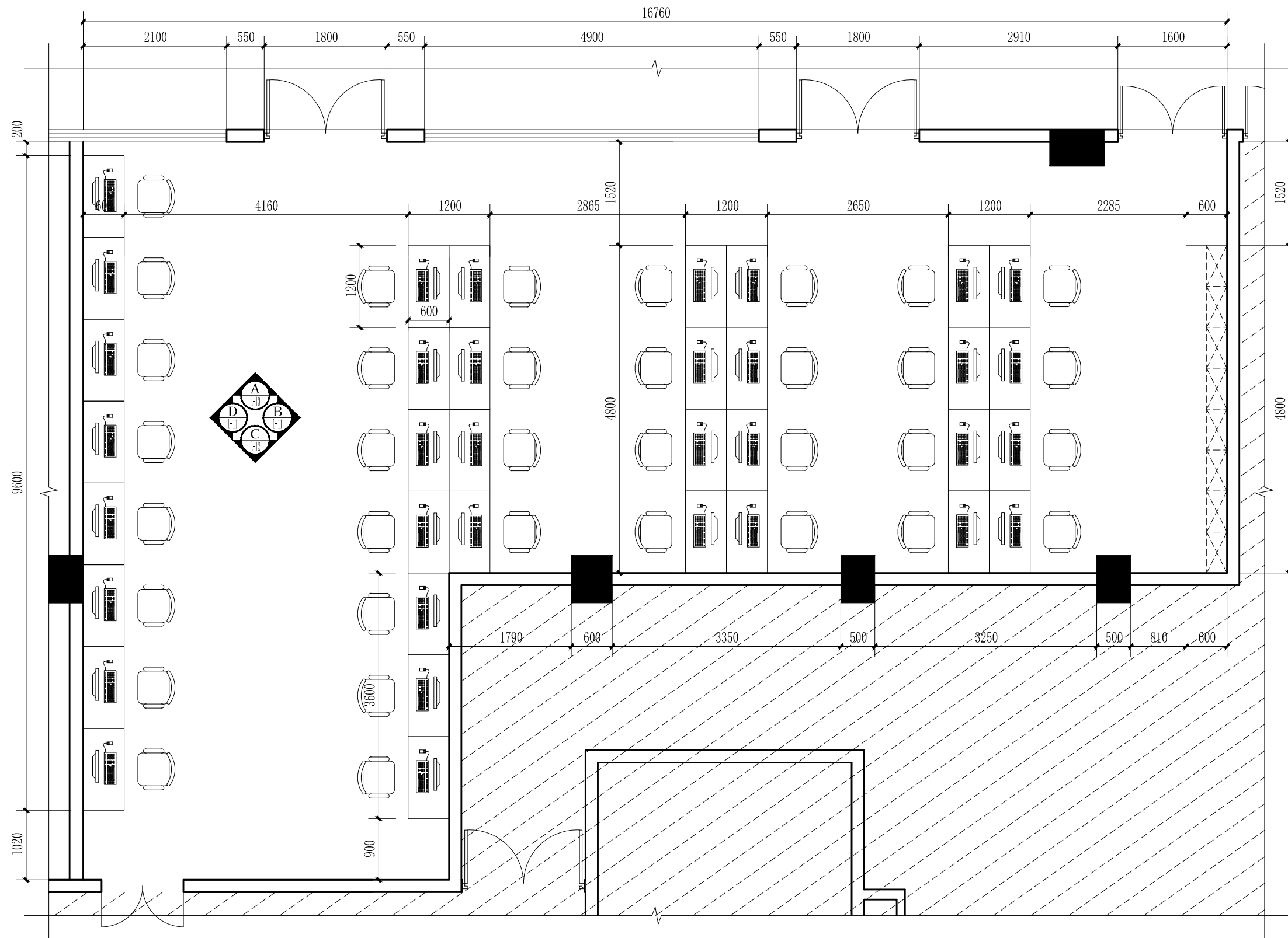
车载监控中心平面图 scale 1:60
