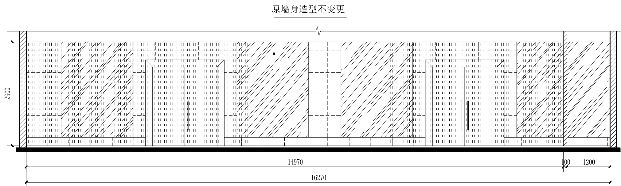
智能调度大厅A立面图scale 1:60
