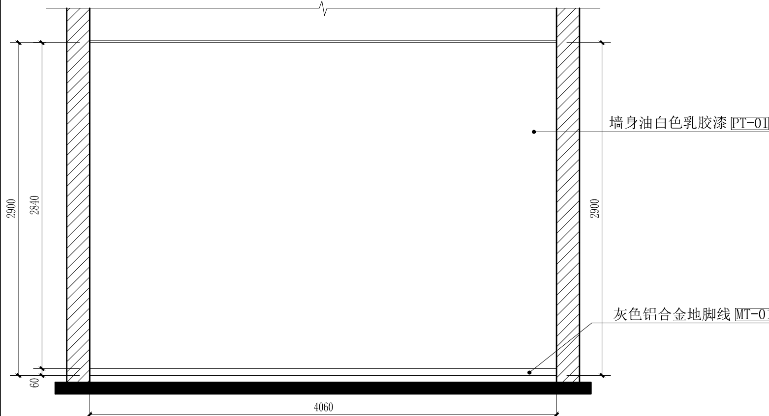
运调监控中心B立面图 scale 1:30
