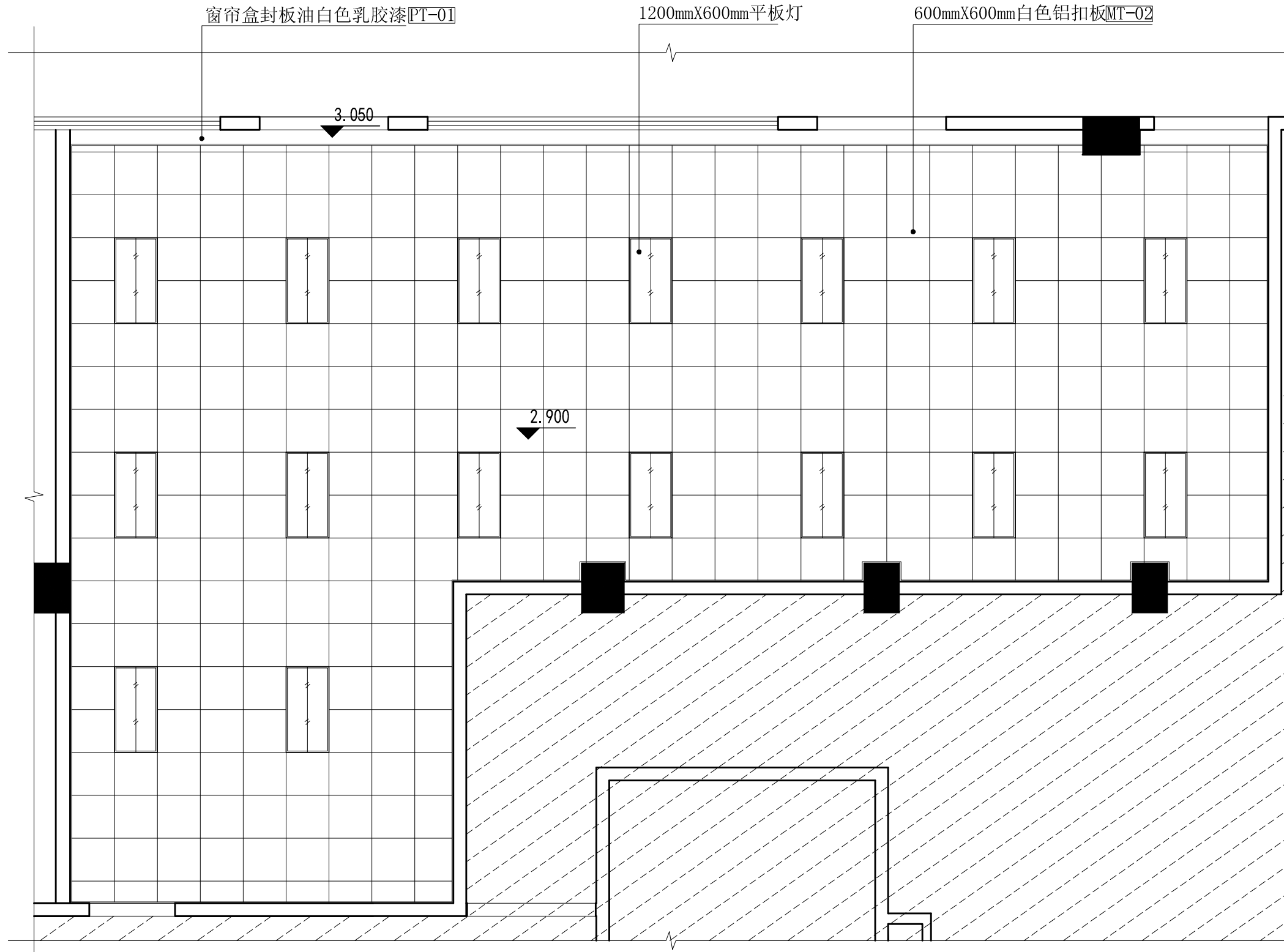
车载监控中心天花图 scale 1:60
