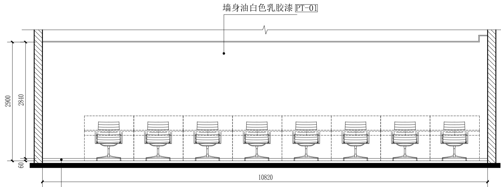
车载监控中心D立面图scale 1:50
