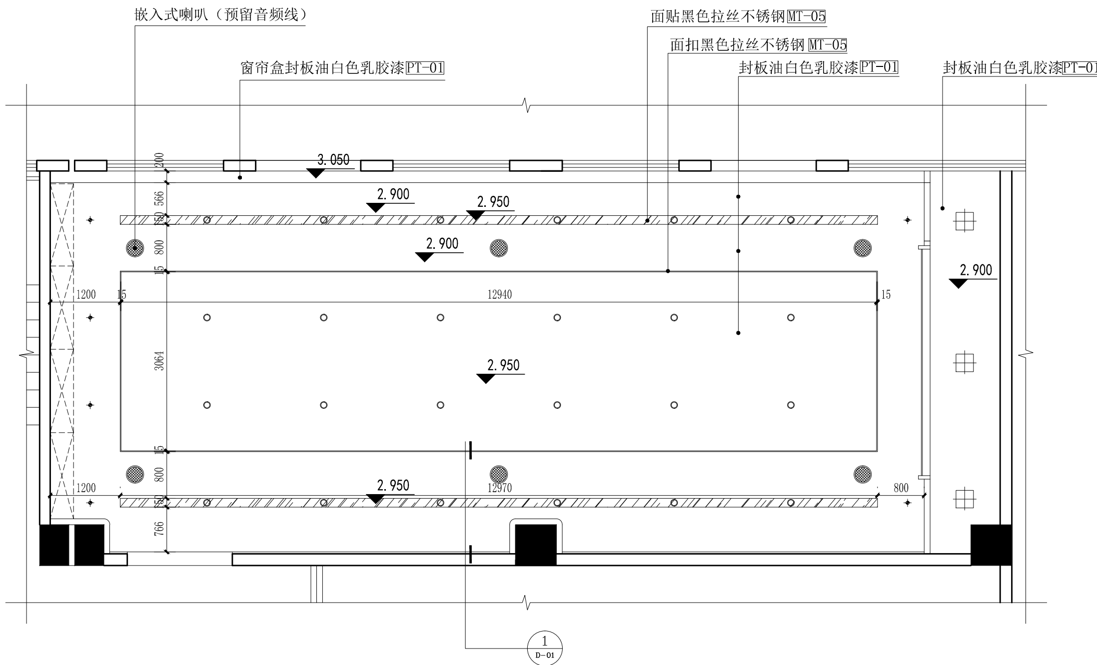
智能调度大厅天花图 scale 1:60
