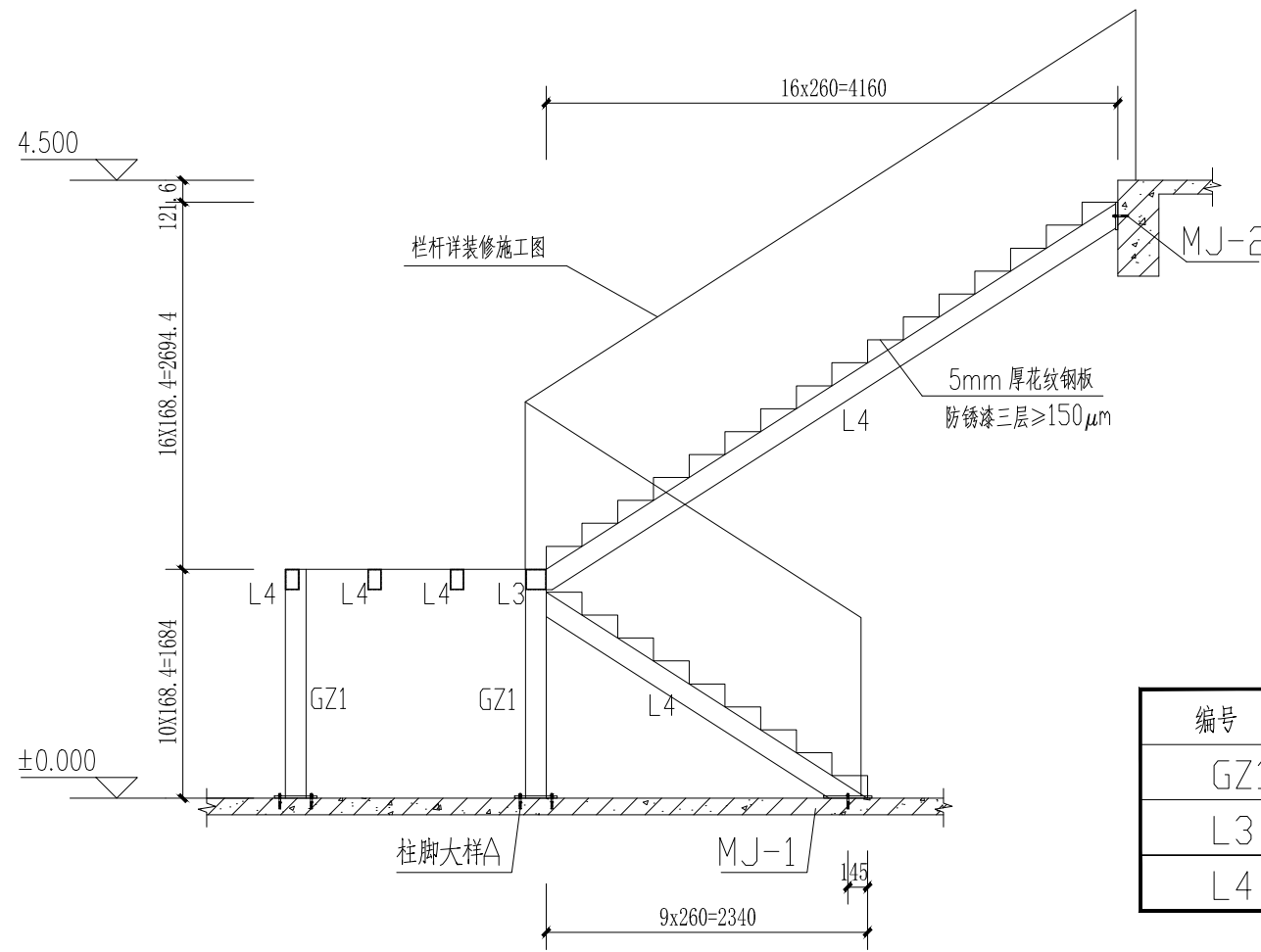
3-3 1:50
