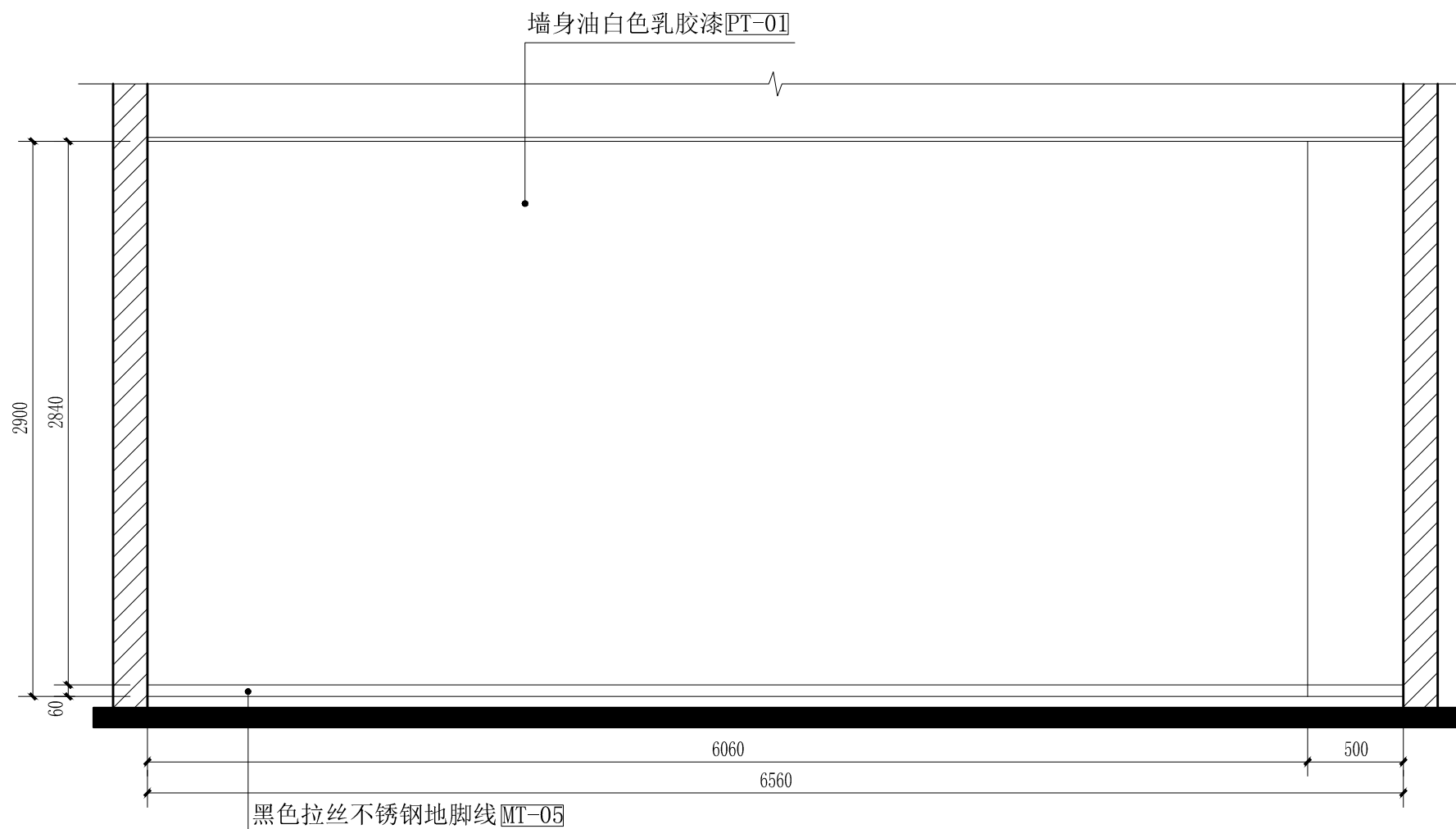
智能调度大厅E立面图 scale 1:30
