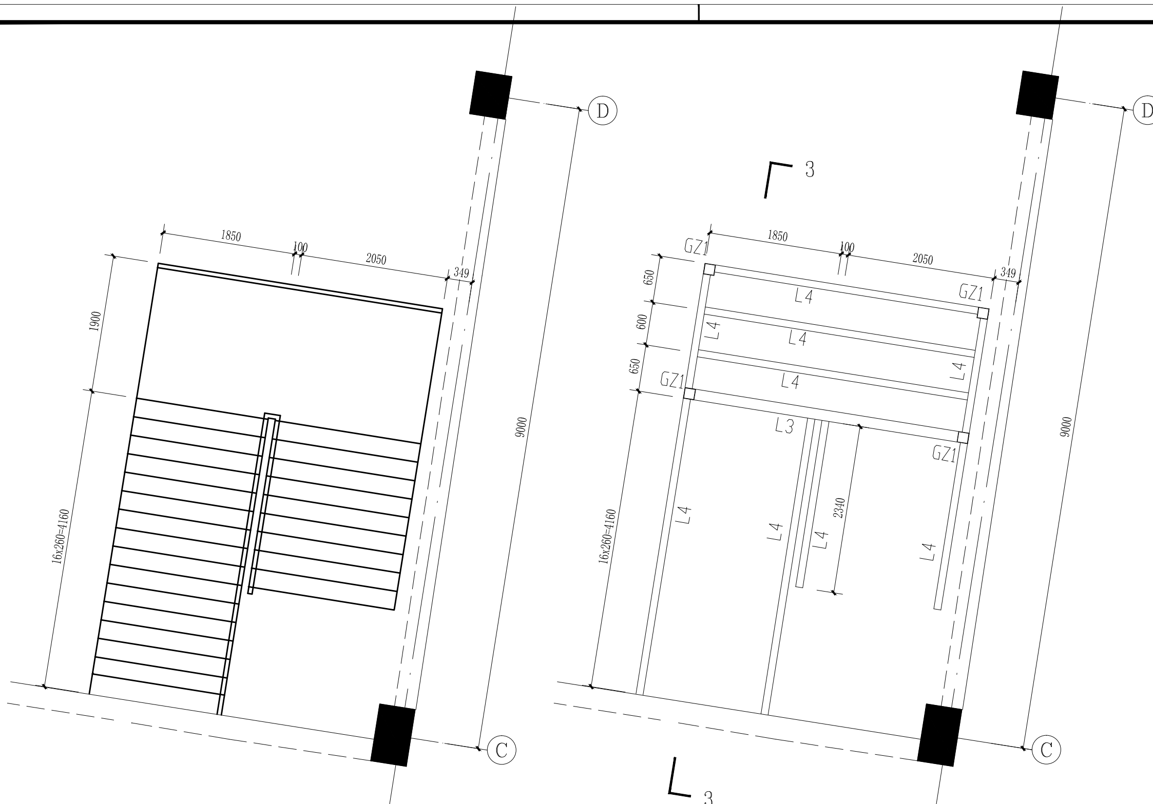
楼梯平面布置图 1:50
