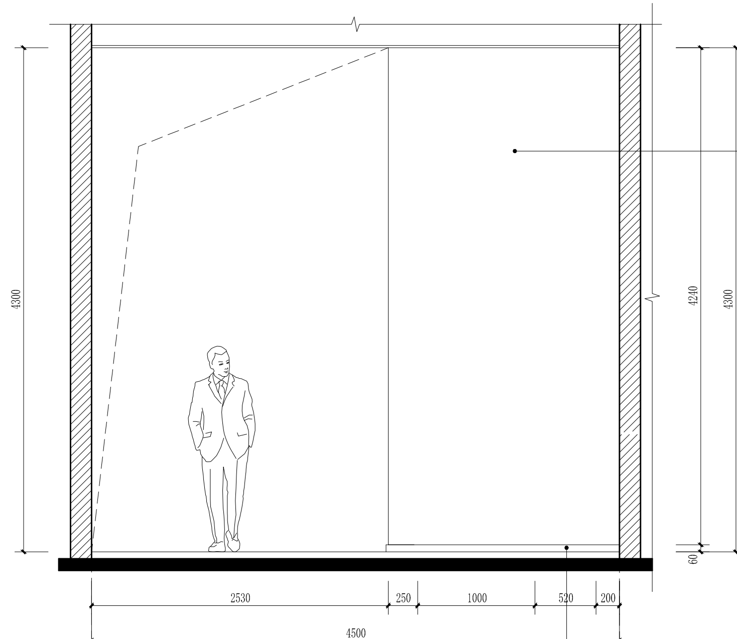
楼梯间 C立面图 scale 1:30
