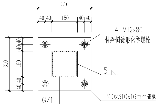
柱脚大样A
