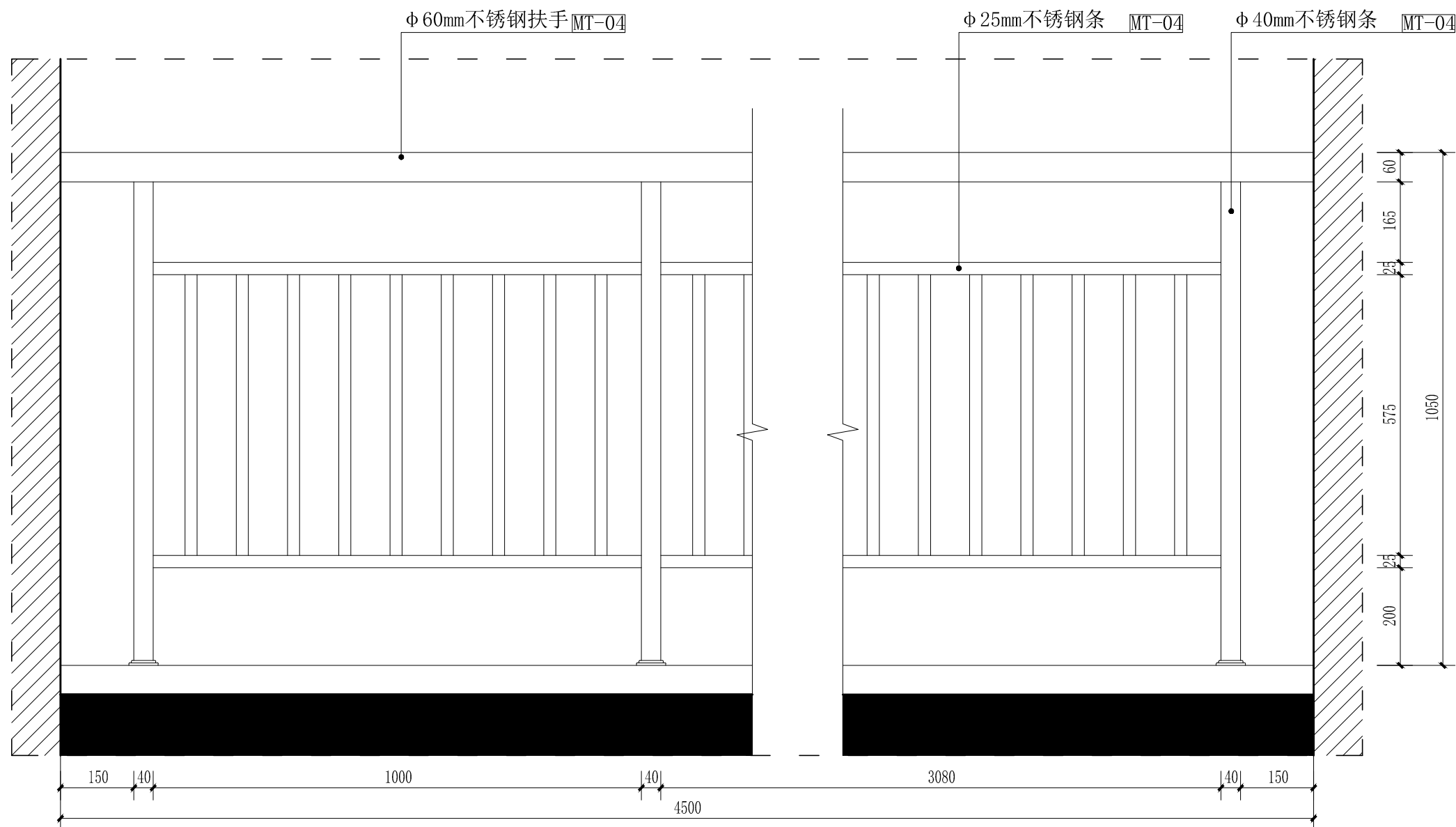
不锈钢拦河立面图 scale 1:15
