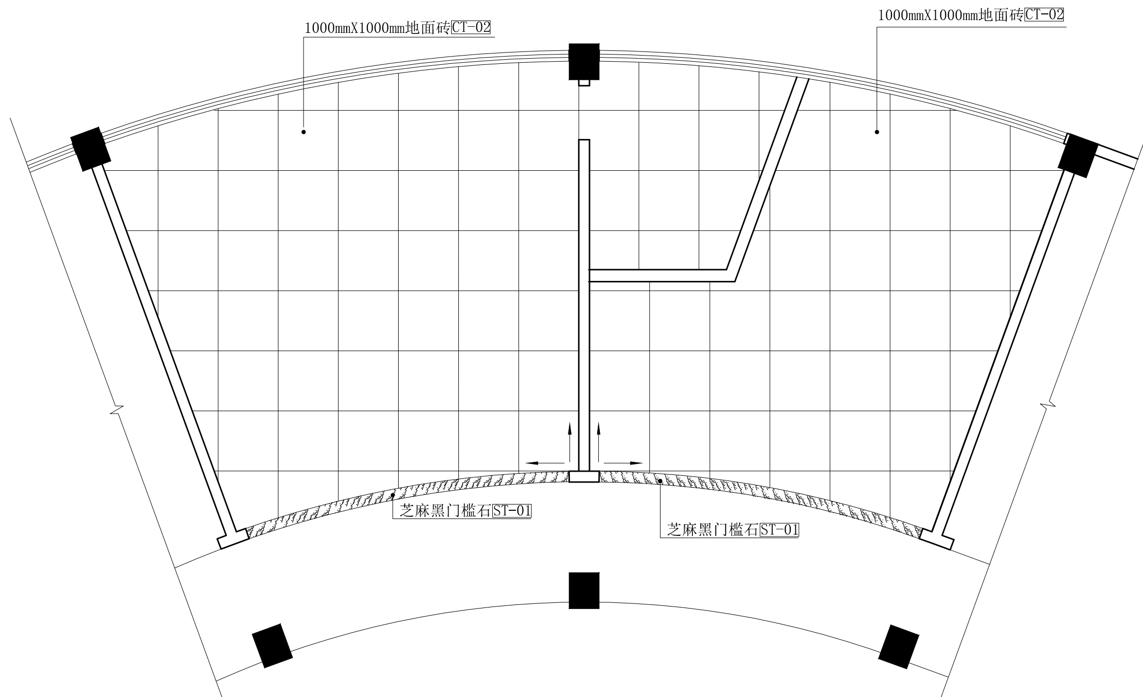
服务热线室、客服服务中心地面铺贴图 scale 1:60
