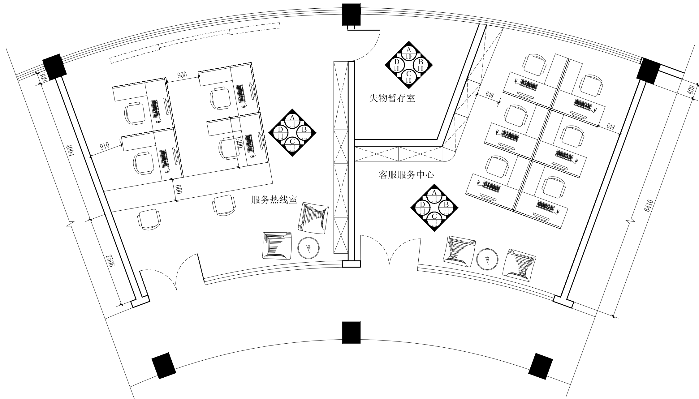
服务热线室、客服服务中心平面图 scale 1:60
