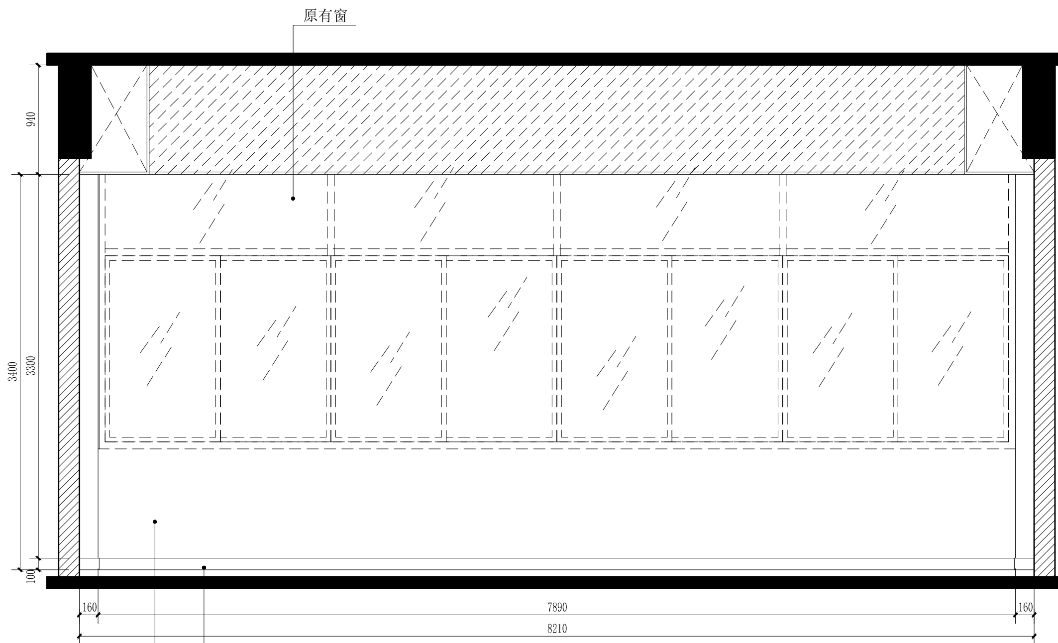
服务热线室A立面图 scale 1:30
