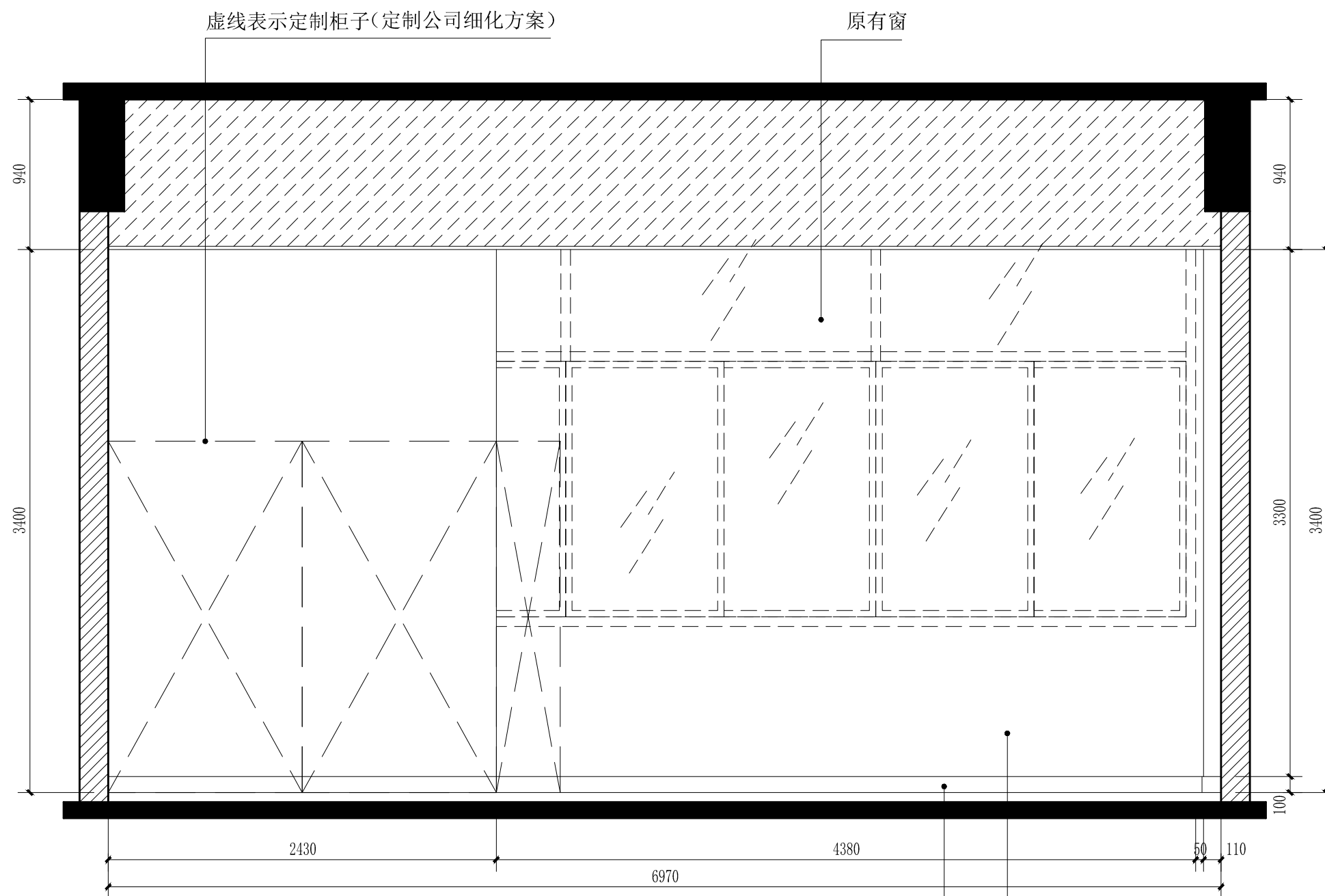
客服服务中心A立面图 scale 1:30
