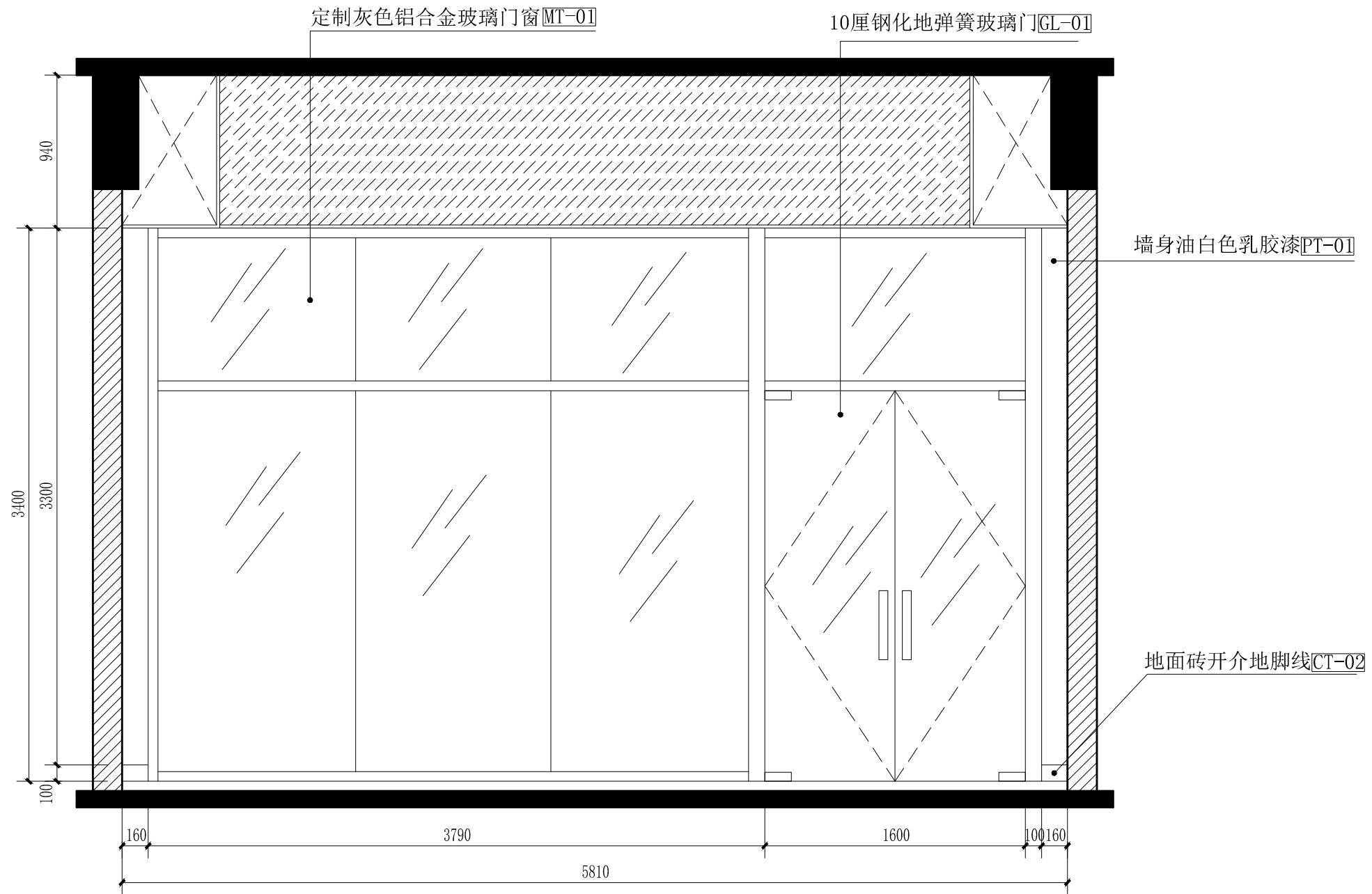
客服服务中心C立面图 scale 1:30
