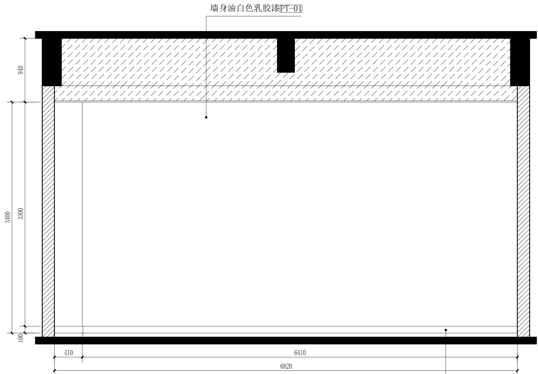
客服服务中心B立面图 scale 1:30
