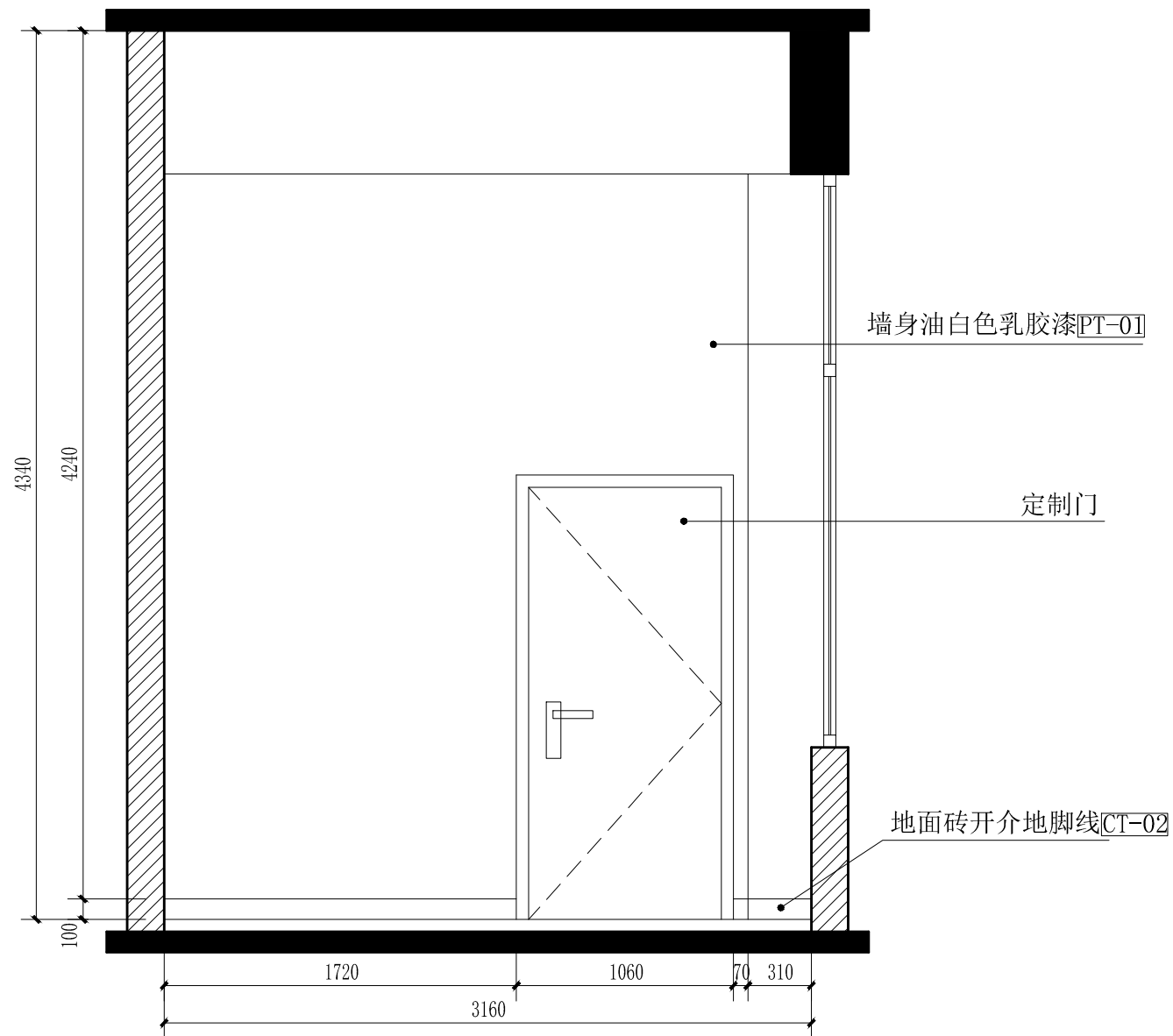
失物暂存室C立面图 scale 1:30
